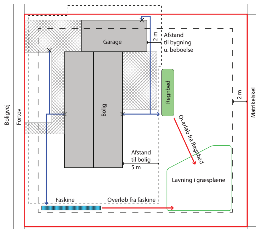
Figur 12: Figuren viser, hvor på grunden det er tilladt at nedsvive regnvand og giver et eksempel på indpasning af en faskine og et regnbed. De røde pile viser, hvilken vej vandet vil strømme, når nedsvivningsanlæggene er overbelastede ved ekstrem nedbør. Illustration Orbicon
