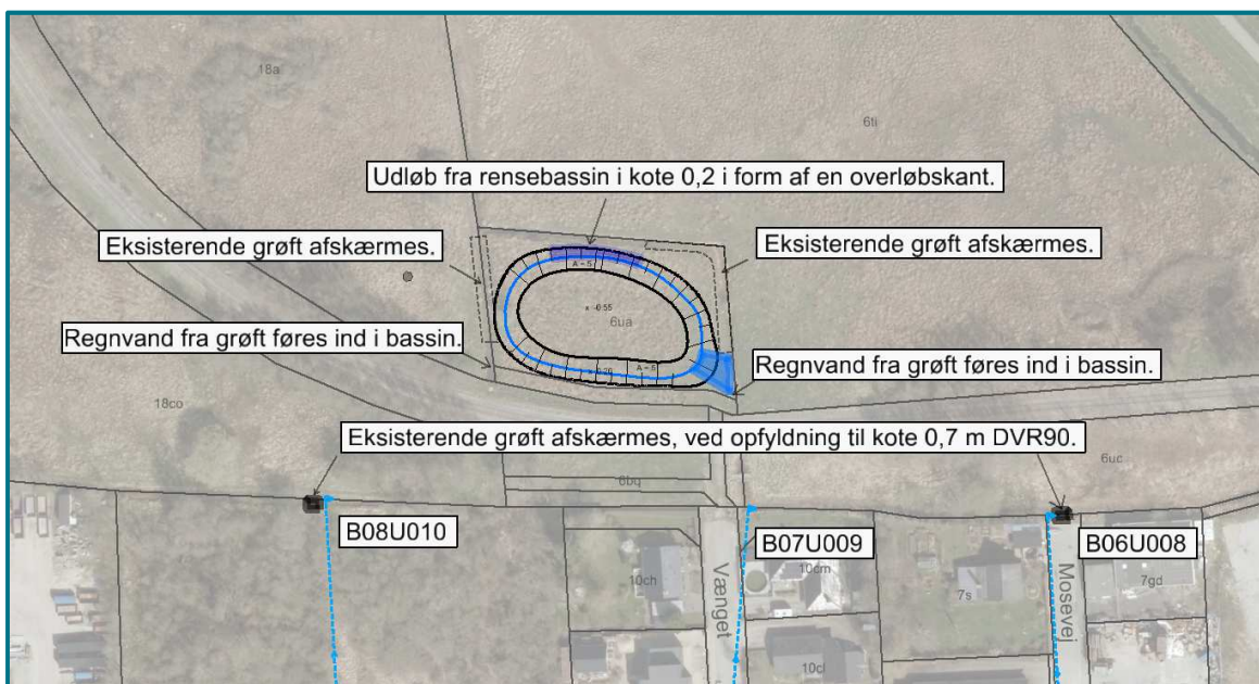
Figur 4. Illustration af anbefalet rensebassin. Mørkblå: udløb i kote 0,2 – Bund i bassin etableres i kote -0,55. Anlæg:1:5.
