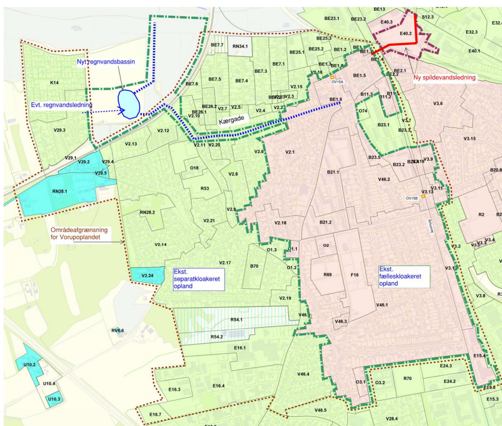
Figur 1. Oplandsoverblik Vorup med afskærende ledning fra kommende separatkloakering (blå stiplet).
