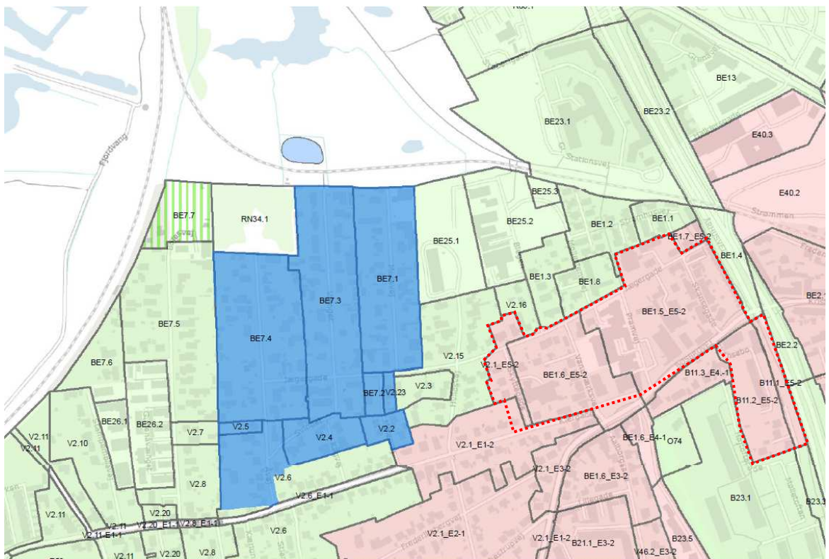
Figur 2. Arealer afgrænset med rød stiplede, angiver oplande, der fremtidigt separatkloakeres med udledning af regnvand til Storkeengen. Oplandsareal fremhævet med blå er separatkloakeret med omtrent samme størrelse og ligger til grund for beregning af renservolumen ved etablering af regnvandsbassin umiddelbart nord for nedlagt jernbane i Storkeengen.
