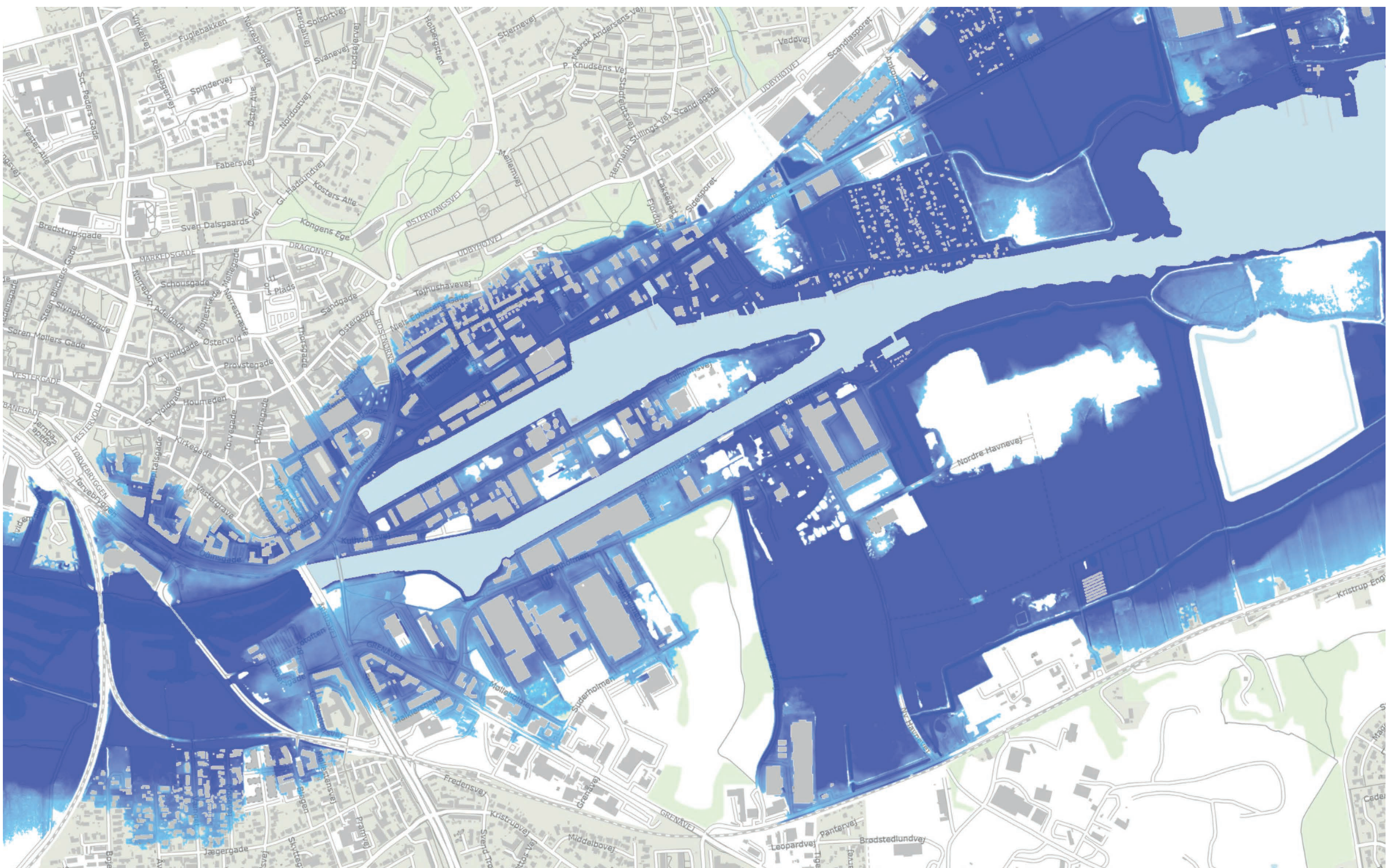
Stormflod kote 2,4 m Uden Klimabåndet og Klimabroen
