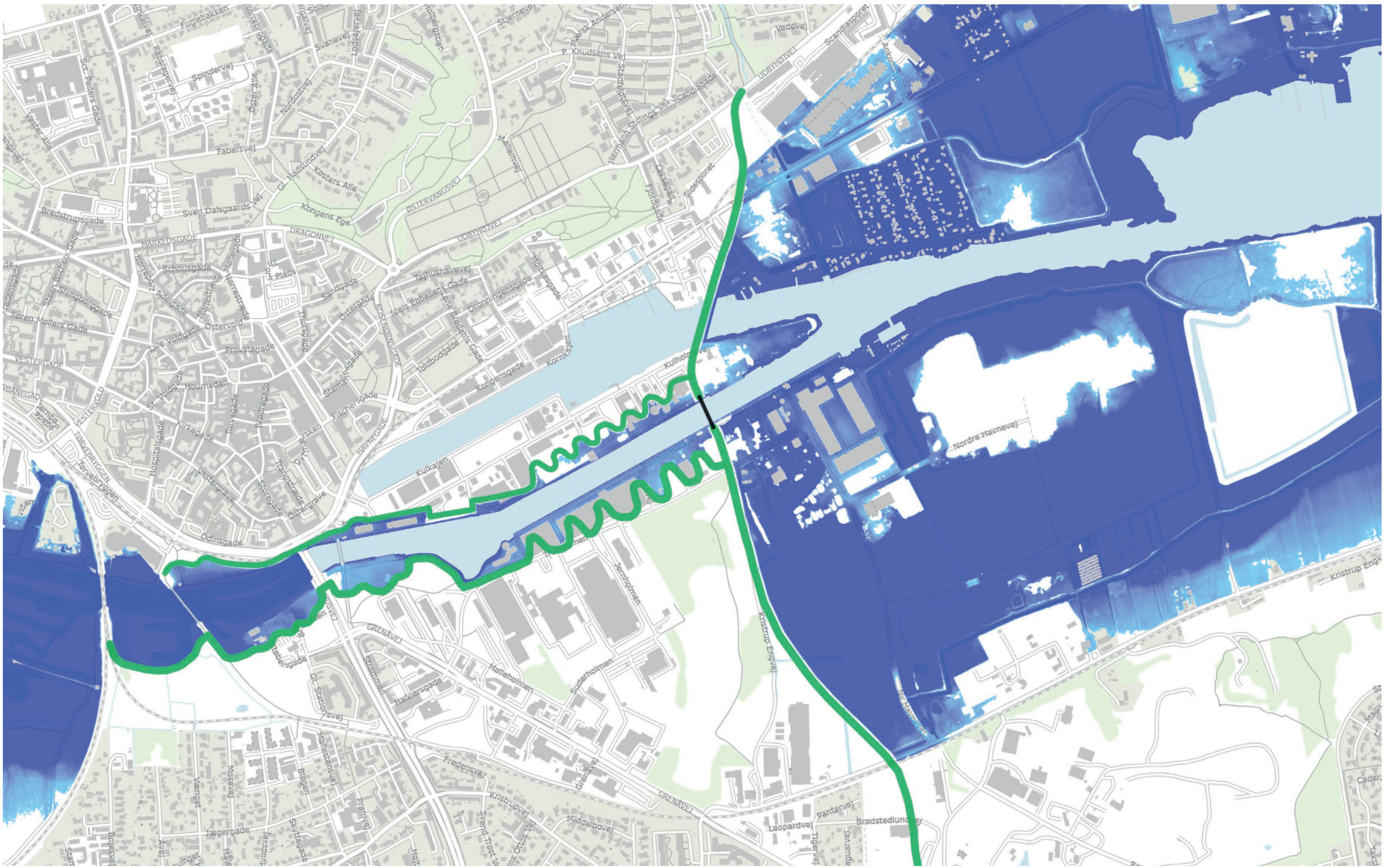
Stormflod kote 2,4 m Med Klimabåndet og Klimabroen
